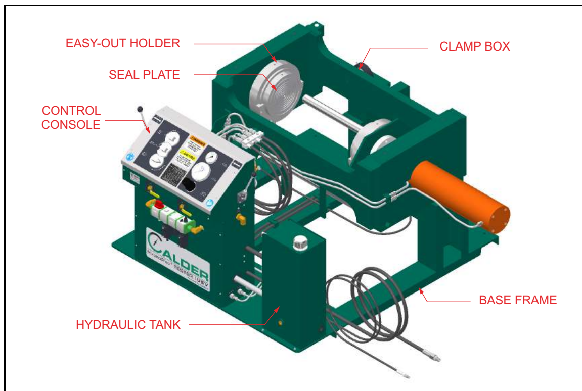
Рисунок 2-1. Компоненты
