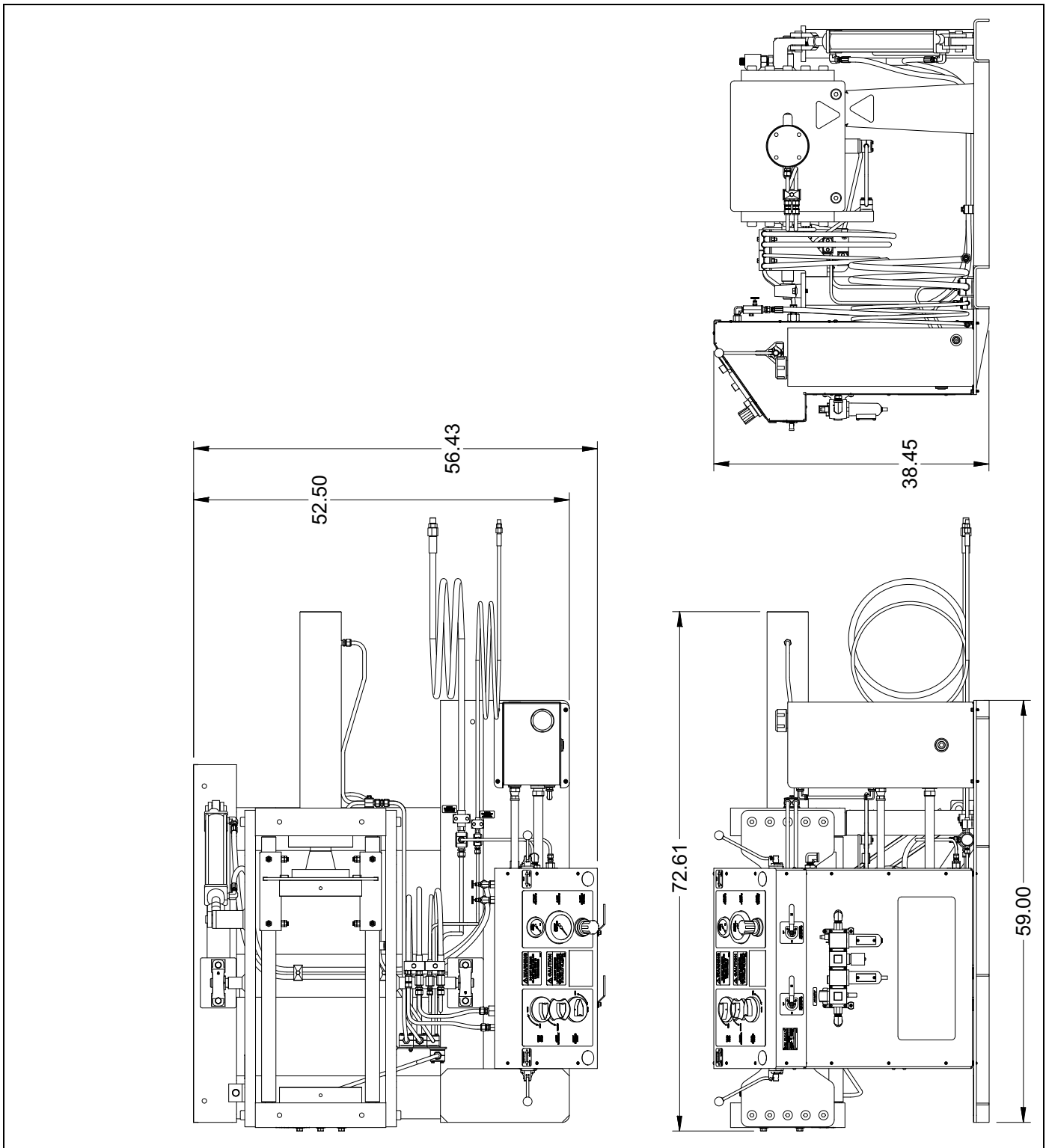
РИСУНОК 2-5. РАЗМЕРЫ ЗАЖИМНОГО ПРИСПОСОБЛЕНИЯ
