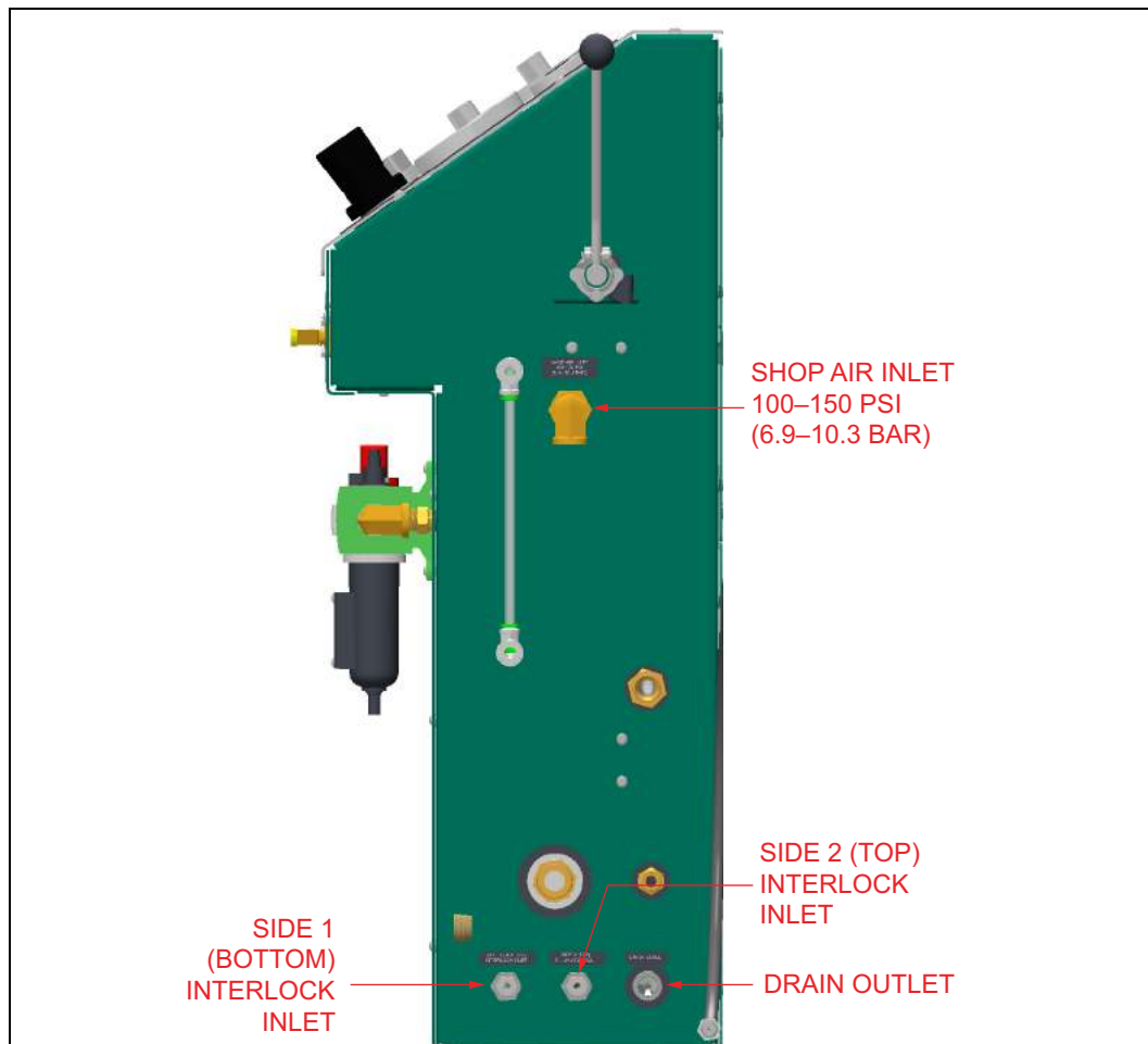
Рисунок 2-4. Управляющие устройства на правой стороне консоли
