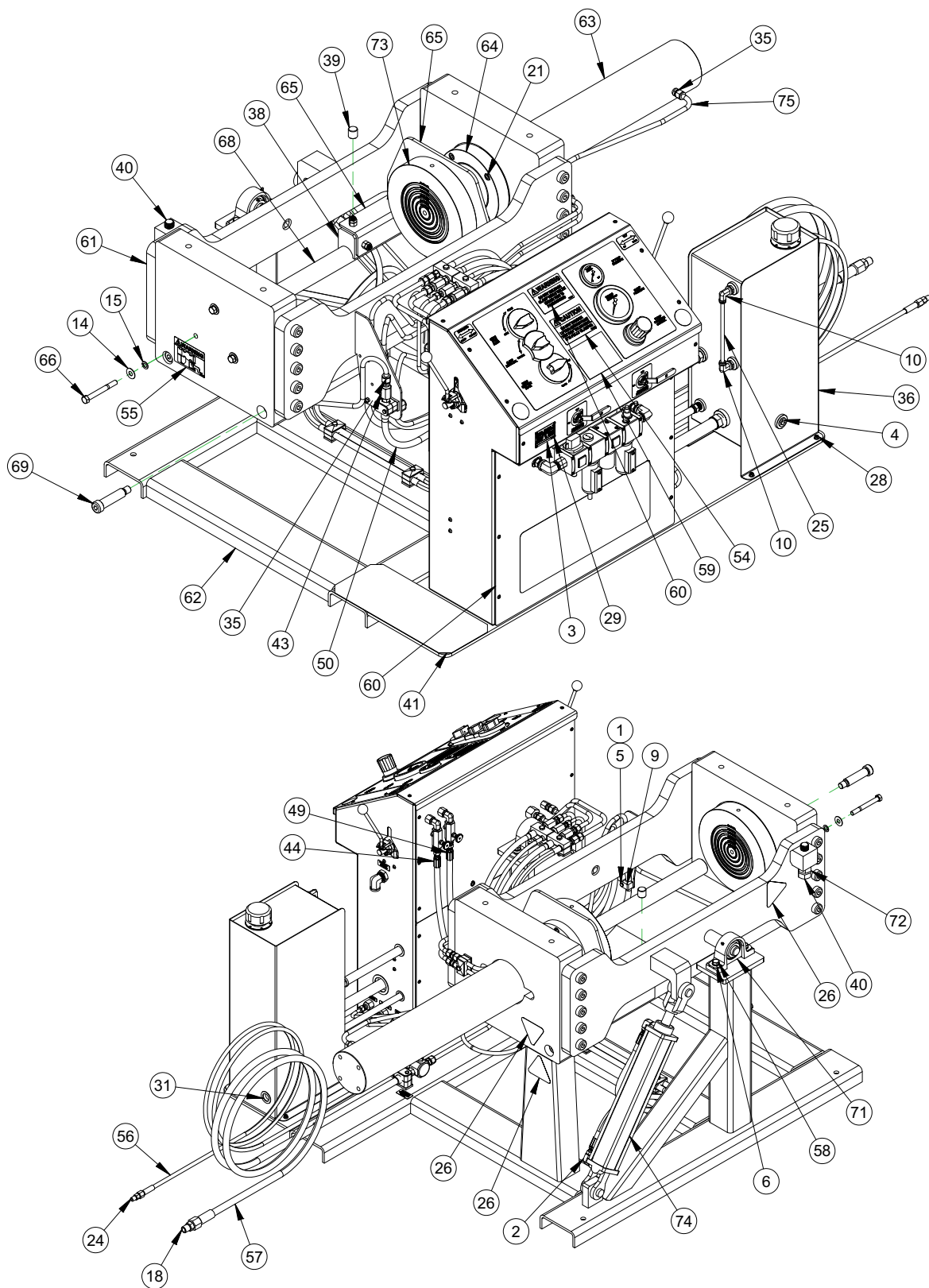
РИСУНОК А-1. USV-6-80Т НАКЛОННОЕ ЗАЖИМНОЕ ПРИСПОСОБЛЕНИЕ В СБОРЕ (P/N 88576)
