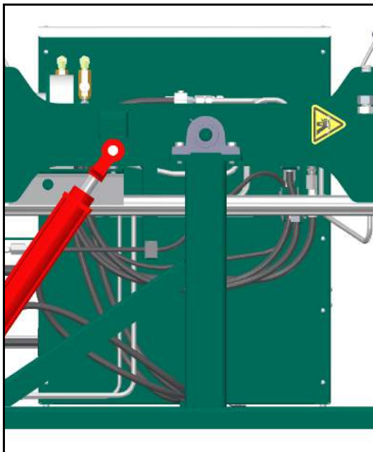
РИСУНОК 1-4. РАСПОЛОЖЕНИЕ МЕТКИ НА ЗАДНЕЙ СТОРОНЕ ЗАЖИМНОГО УСТРОЙСТВА
