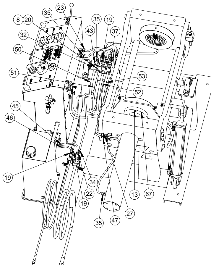
РИСУНОК А-2. USV-6-80Т НАКЛОННОЕ ЗАЖИМНОЕ ПРИСПОСОБЛЕНИЕ В СБОРЕ 2 (P/N 88576)
