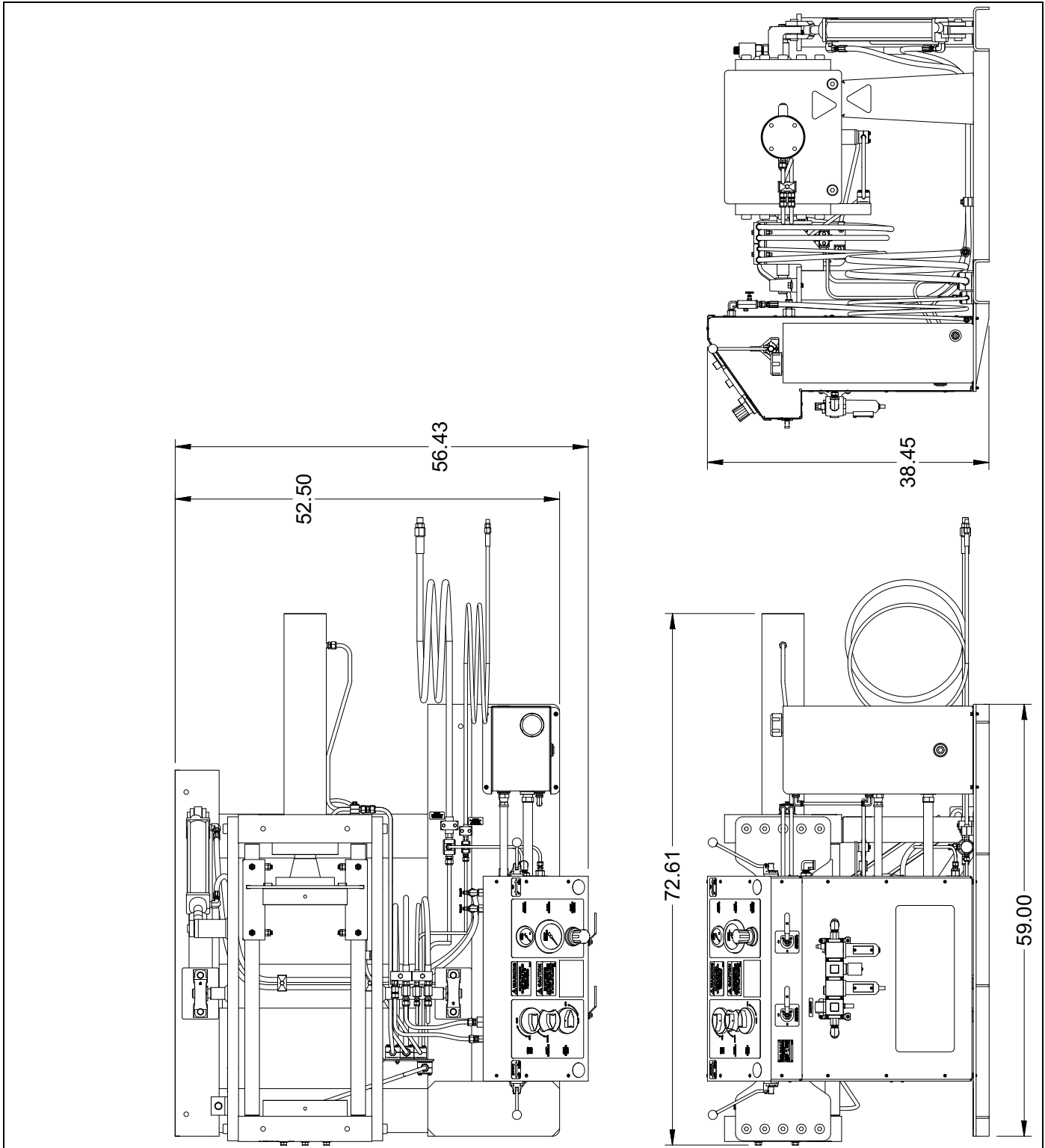
FIGURE 2-5. DIMENSIONS DU SYSTÈME DE SERRAGE
