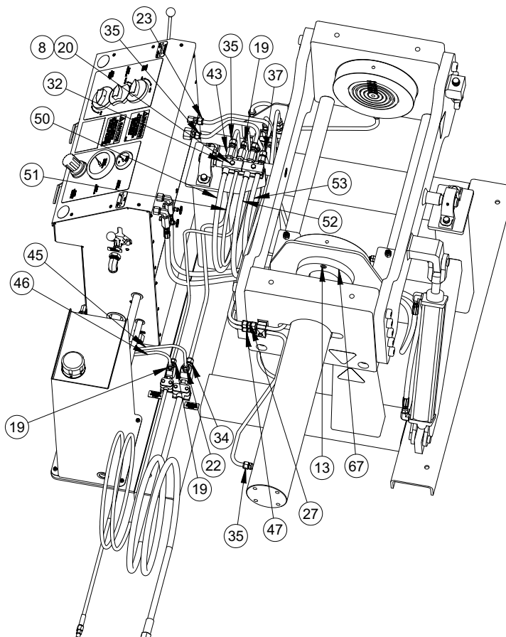
FIGURE A-2. USV-6-80T D'INCLINAISON ENSEMBLE SYSTÈME DE SERRAGE 2 (P/N 88576)
