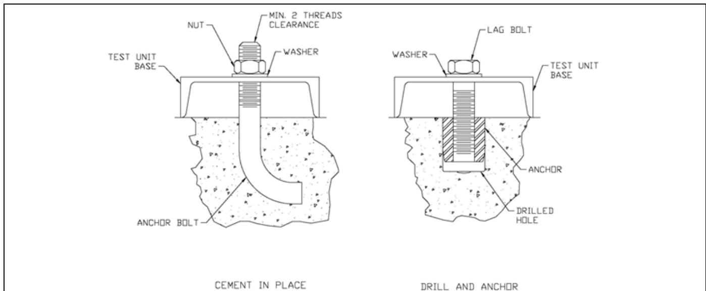
РИСУНОК 3-1. ФИКСАЦИЯ ИСПЫТАТЕЛЬНОГО СТЕНДА
