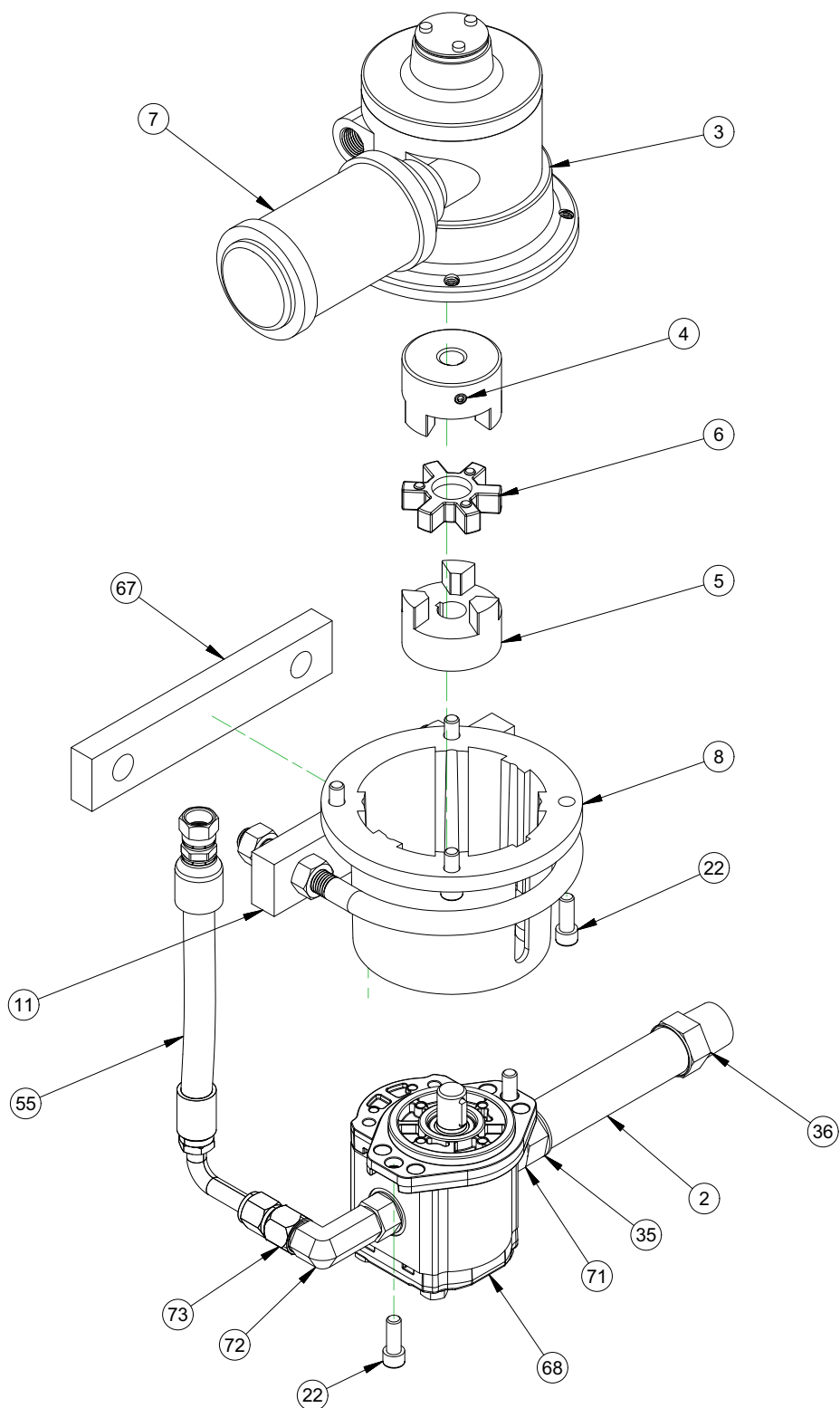
Рисунок А-8. USV-12-150Т ДЕТАЛЬНЫЙ ВИД НАСОСА НИЗКОГО ДАВЛЕНИЯ (P/N 87922)
