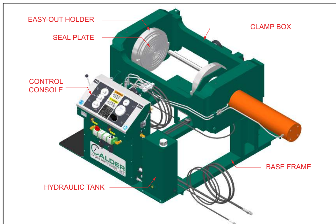
ABBILDUNG 2-1. KOMPONENTEN
