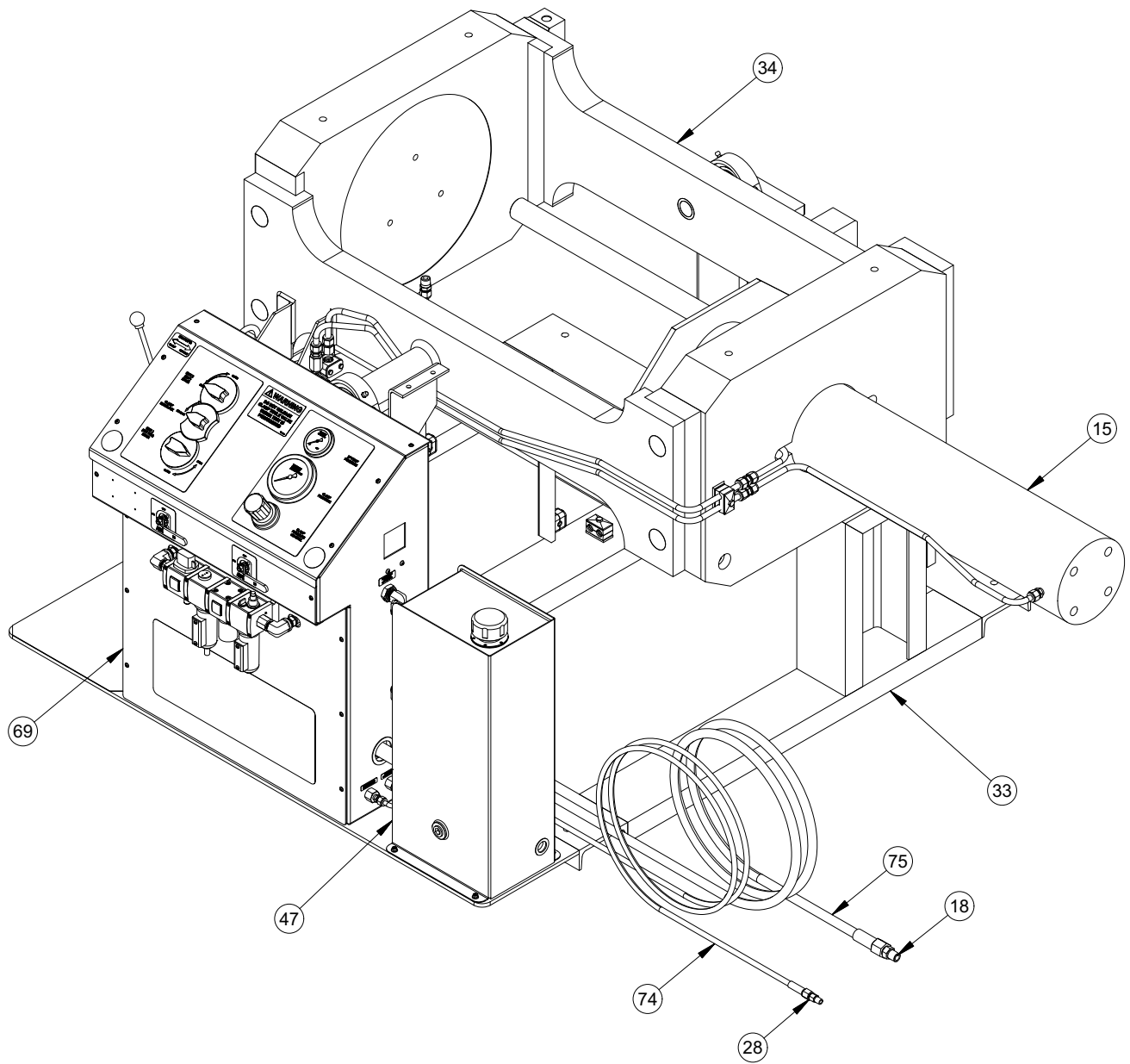
ABBILDUNG A-6. USV-12-150T BAUTEILELISTE 1 (P/N 87992)
