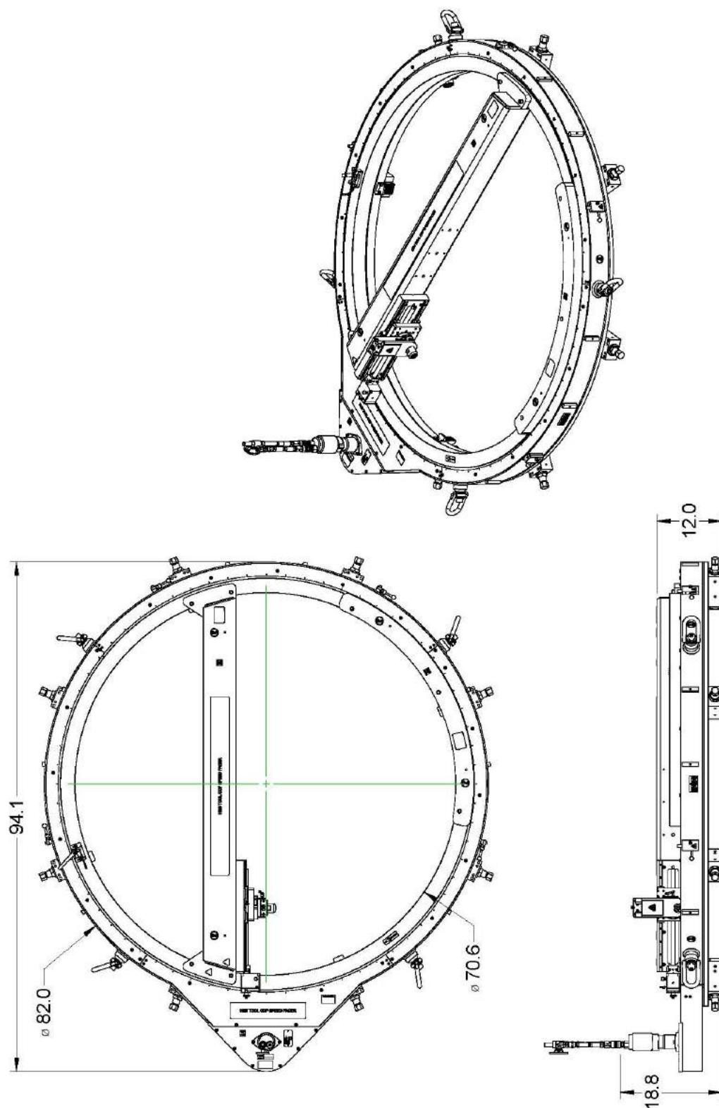
ABBILDUNG 2-3. ODF70 FLANSCHDREHMASCHINE ABMESSUNGEN (P/N 87000)
