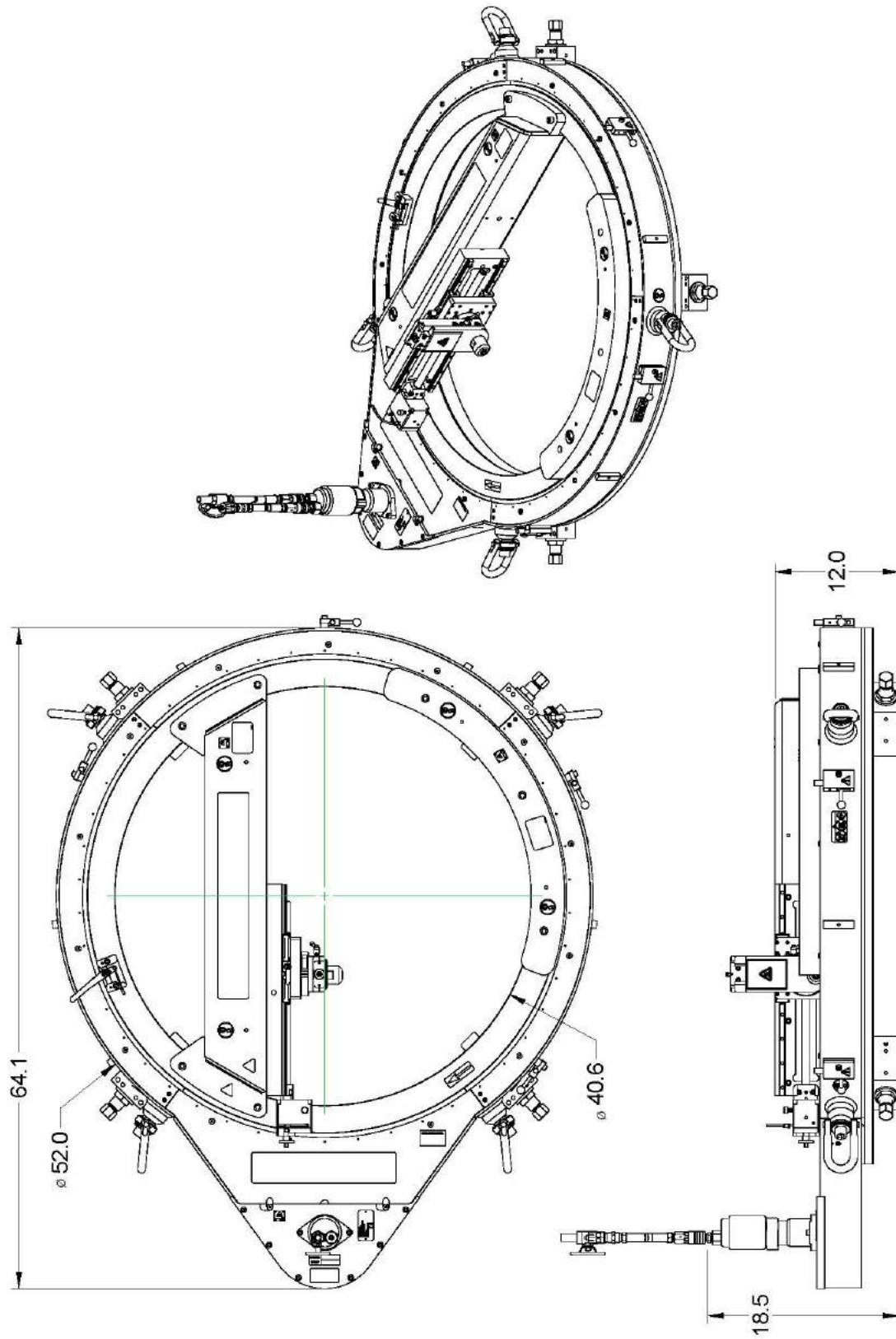
FIGURA 2-3. DIMENSIONES DE LA REFRENTADORA RÁPIDA ODF40 (P/N 86870)
