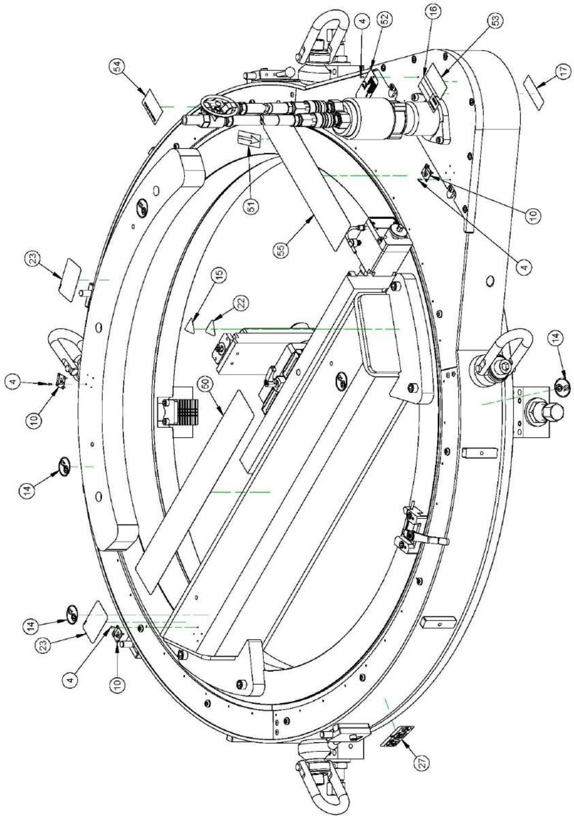
FIGURA A-2. MONTAJE DE LAS ETIQUETAS DE LA REFRENTADORA RÁPIDA ODF40 (P/N 86870)
