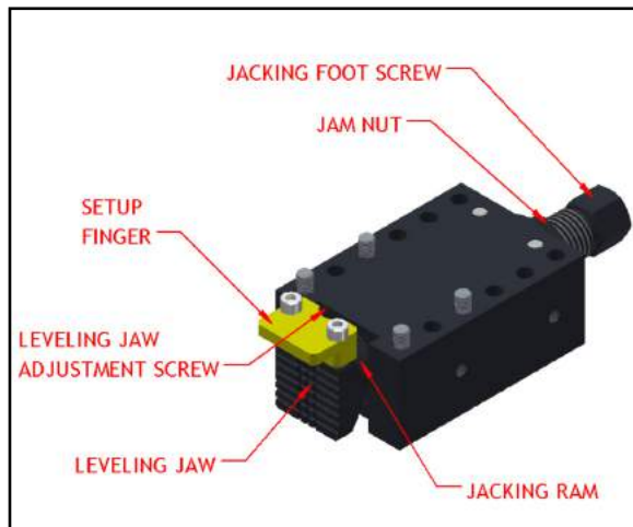
FIGURA 3-6. COMPONENTES DE LA PATA REGULABLE
