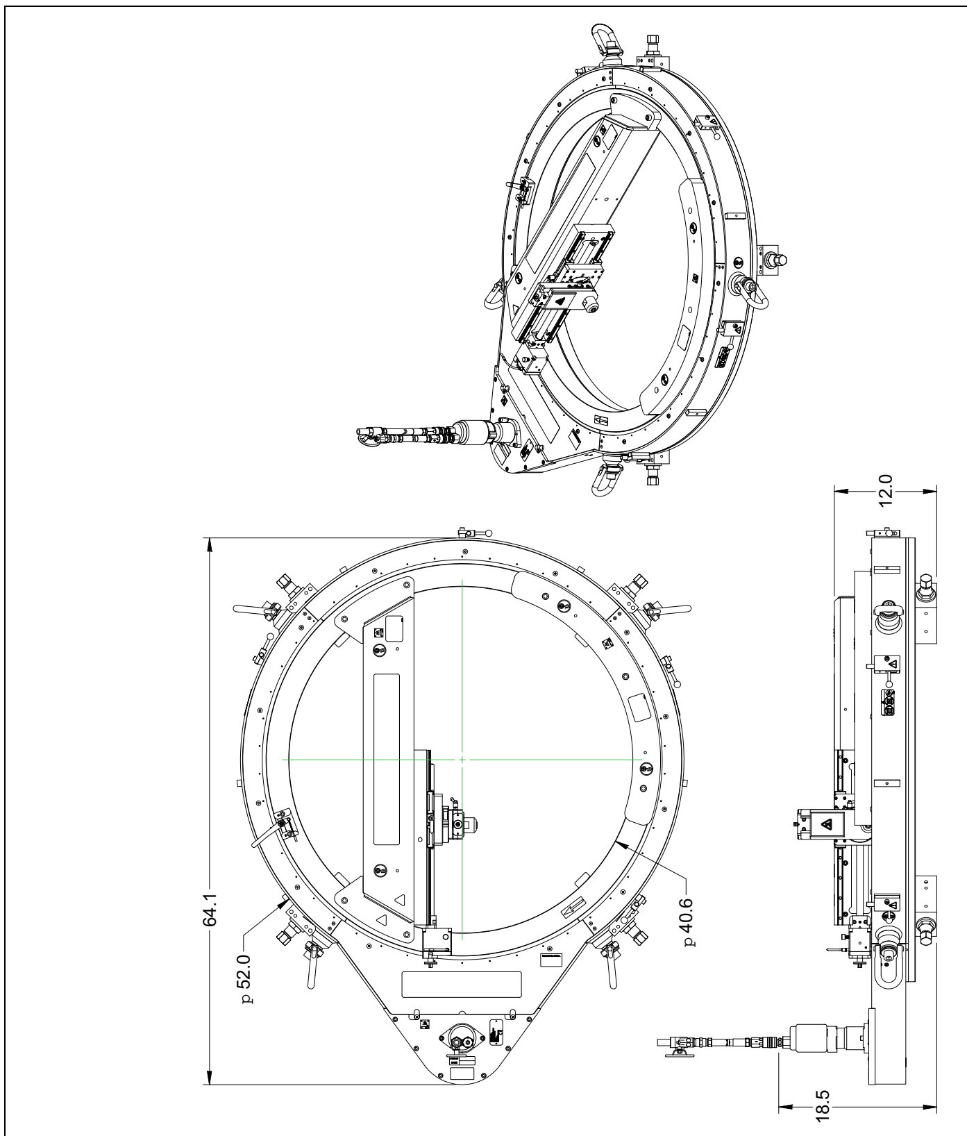
РИСУНОК 2-3. РАЗМЕРЫ ODF40 SPEED FACER (№ ИЗДЕЛИЯ 86870)
