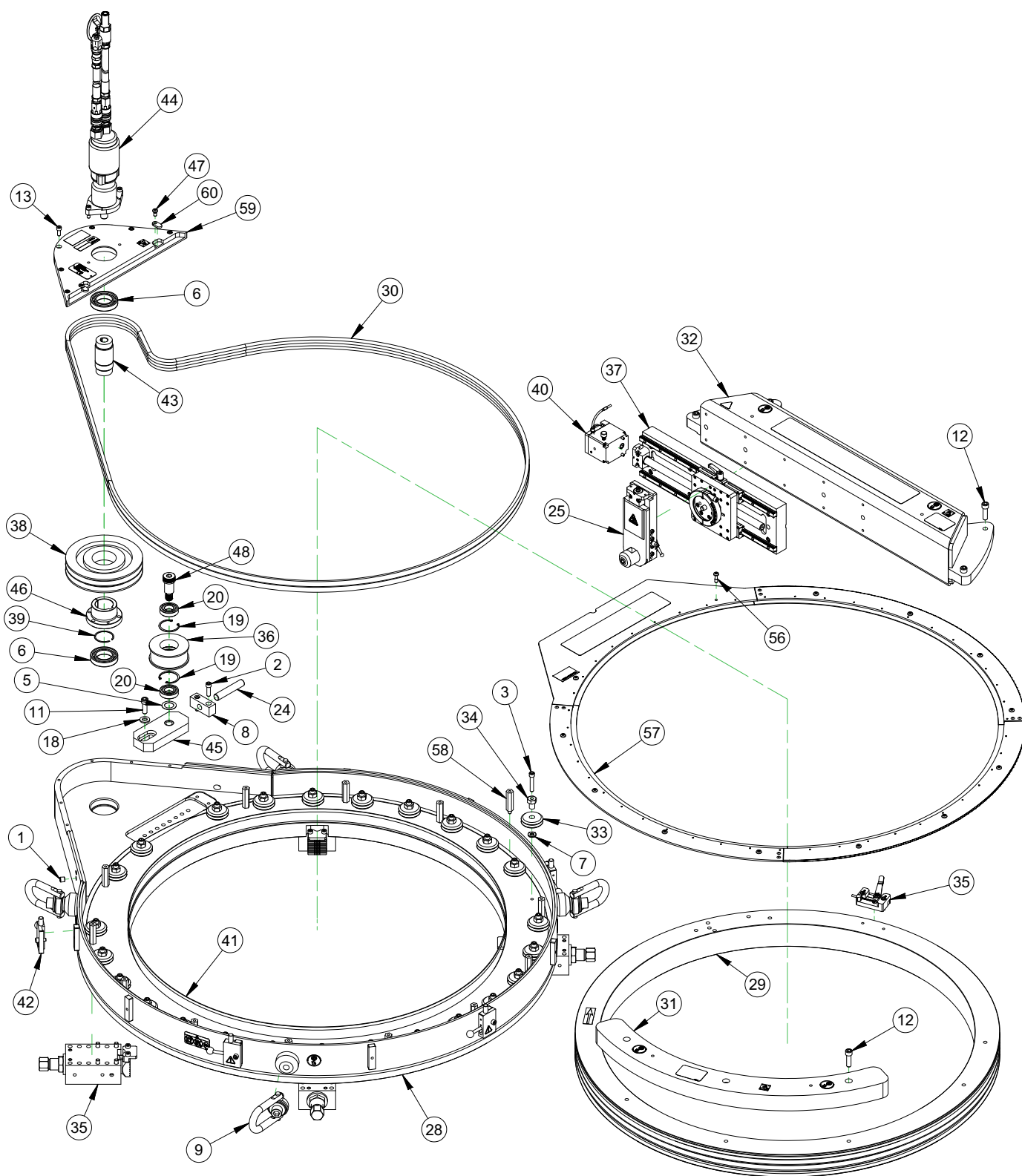
РИСУНОК А-1. ODF40 SPEED FACER В СБОРЕ (№ изделия 86870)
